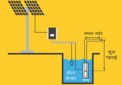
सबमर्सिबल पम्प रेखाचित्र
