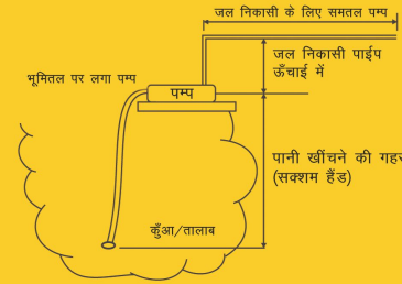
सतहीय पम्प रेखाचित्र
